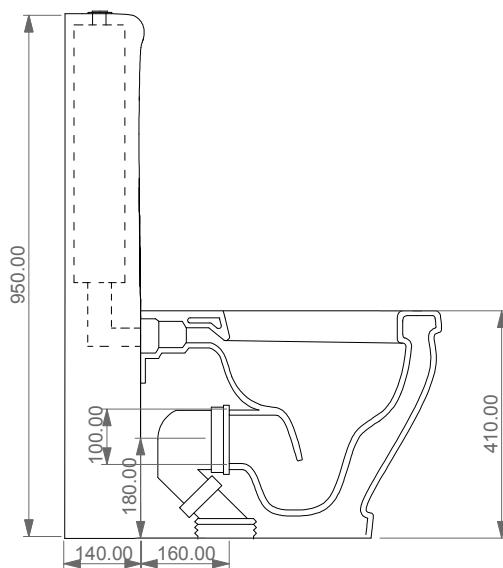
Con connessione eccentrica per scarico a suolo. ACS 102 With outlying drainage connector for floor trap. ACS 102
