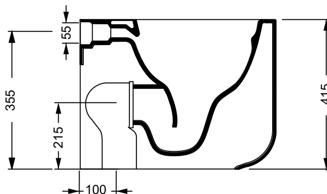
Con connessione per scarico a suolo. ACS 100 With drainage connector for floor trap. ACS 100
