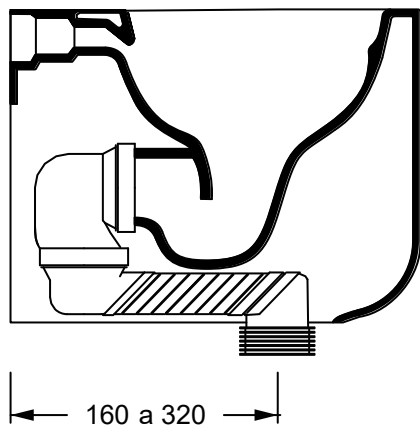
Raccordo piatto per wc Petra. ACS 107 Flat adjustable wc connector for Petra. ACS 107
