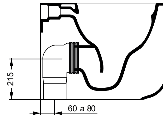
Con connessione per scarico a suolo regolabile. ACS 103 With adjustable drainage connector for floor trap. ACS 103
