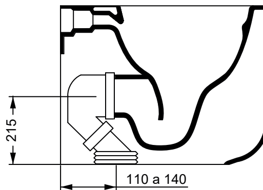
Con connessione traslata per scarico a suolo. ACS 102 With outlying drainage connector for floor trap. ACS 102
