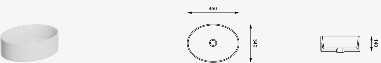
cod. LKLAVFSBF45 Lavabo Like da appoggio o su colonna cm. 45 Countertop or on Pedestal Washbasin Like cm. 45
