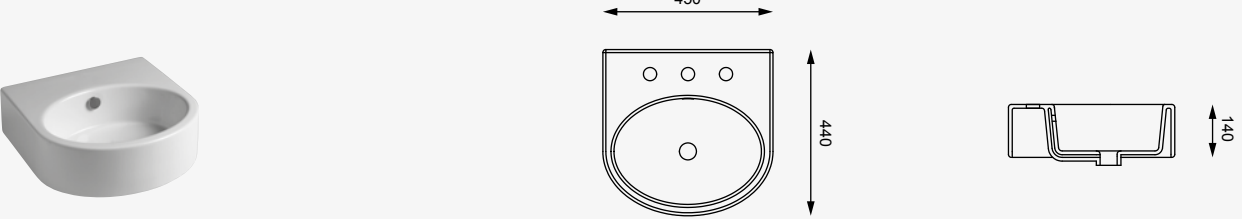
cod. LKLAVBW45 Lavabo Like da appoggio, sospeso o su colonna cm. 45 Countertop, wall-hung or on Pedestal Washbasin Like cm. 45
