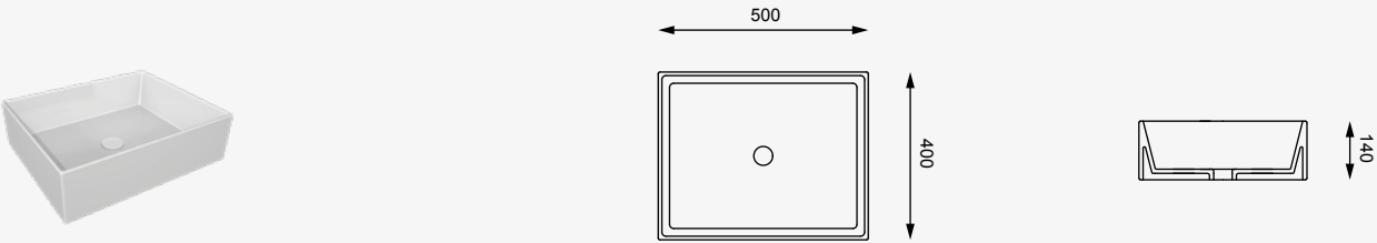
cod. ZELAVFS50 Lavabo da appoggio centro stanza Zenith cm. 50 Countertop free standing Washbasin Zenith cm. 50
