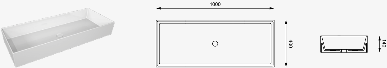
cod. ZELAVFS100 Lavabo da appoggio centro stanza Zenith cm. 100 Countertop free standing Washbasin Zenith cm. 100
