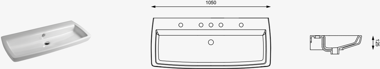
cod. BRLAV105 Lavabo Brio da appoggio o sospeso cm. 105 Countertop or wall-hung washbasin Brio cm. 105
