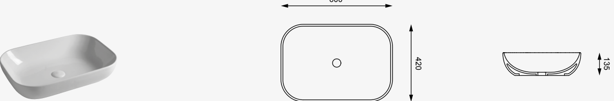
cod. EALAVRE60 Lavabo Easy Rettangolare cm. 60 Easy Washbasin Rectangular cm. 60
