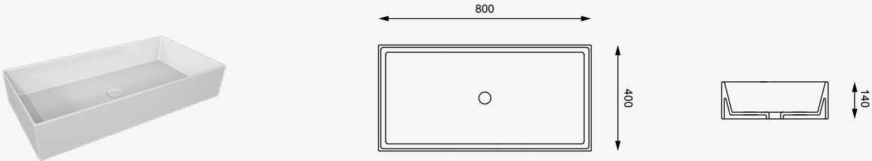
cod. ZELAVFS80 Lavabo da appoggio centro stanza Zenith cm. 80 Countertop free standing Washbasin Zenith cm. 80
